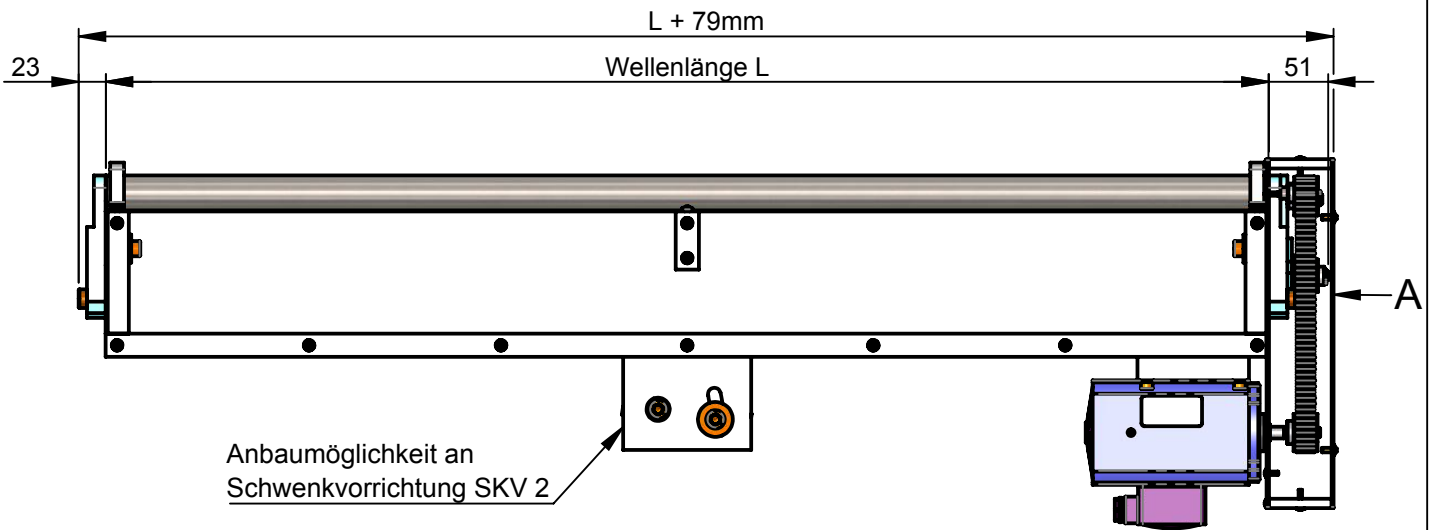
Ansicht A
