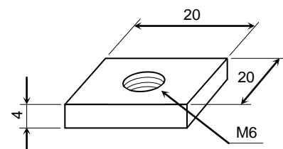
Gewindeplatte E-Nut B.Nr.: 1.31.EM6 (Maytec)
