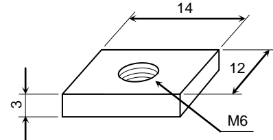
Gewindeplatte F-Nut B.Nr.: 1.31.FM6 (Maytec)
